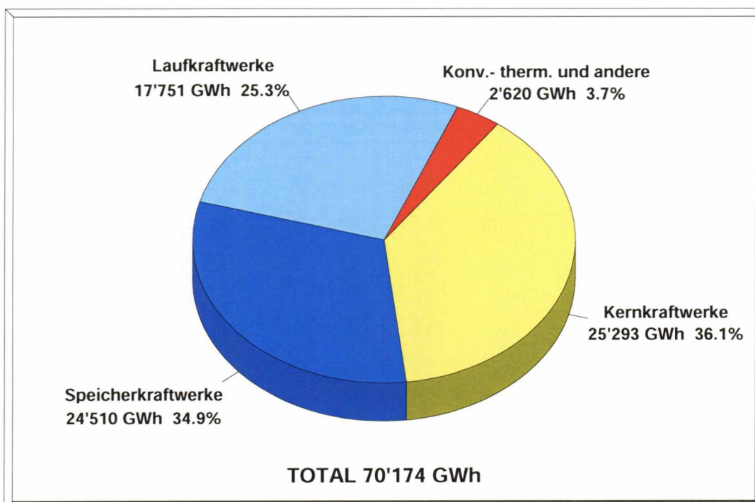
Graphik 1: Produktionsanteile von Elektrizität in der Schweiz im Jahr 2001 (Quelle: Schweiz. Elektrizitätsstatistik)
